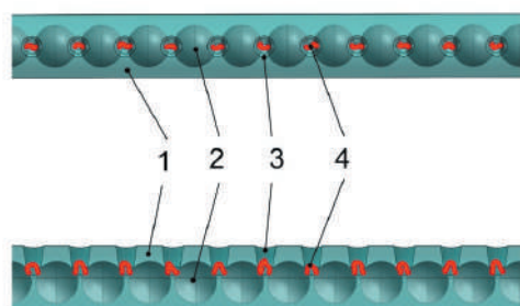
а) схема, поясняющая начальный момент развития разрядов
